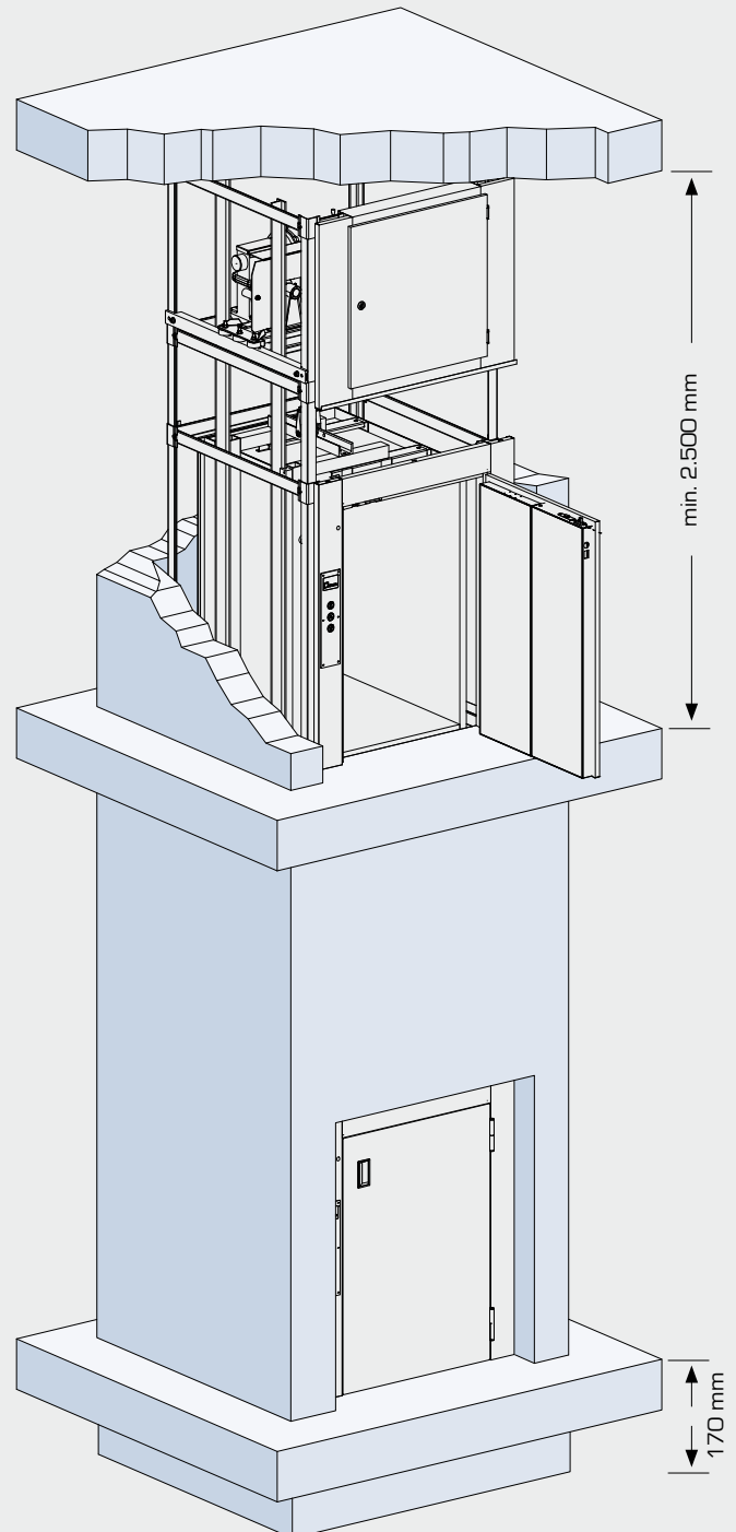
Schnittzeichnung Cargo-Master
